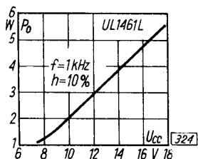
Moc wyjściowa w funkcji napięcia zasilania
