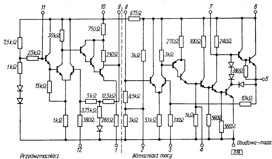
Schemat elektryczny
