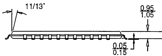
44-Pin TQFP (F44)
