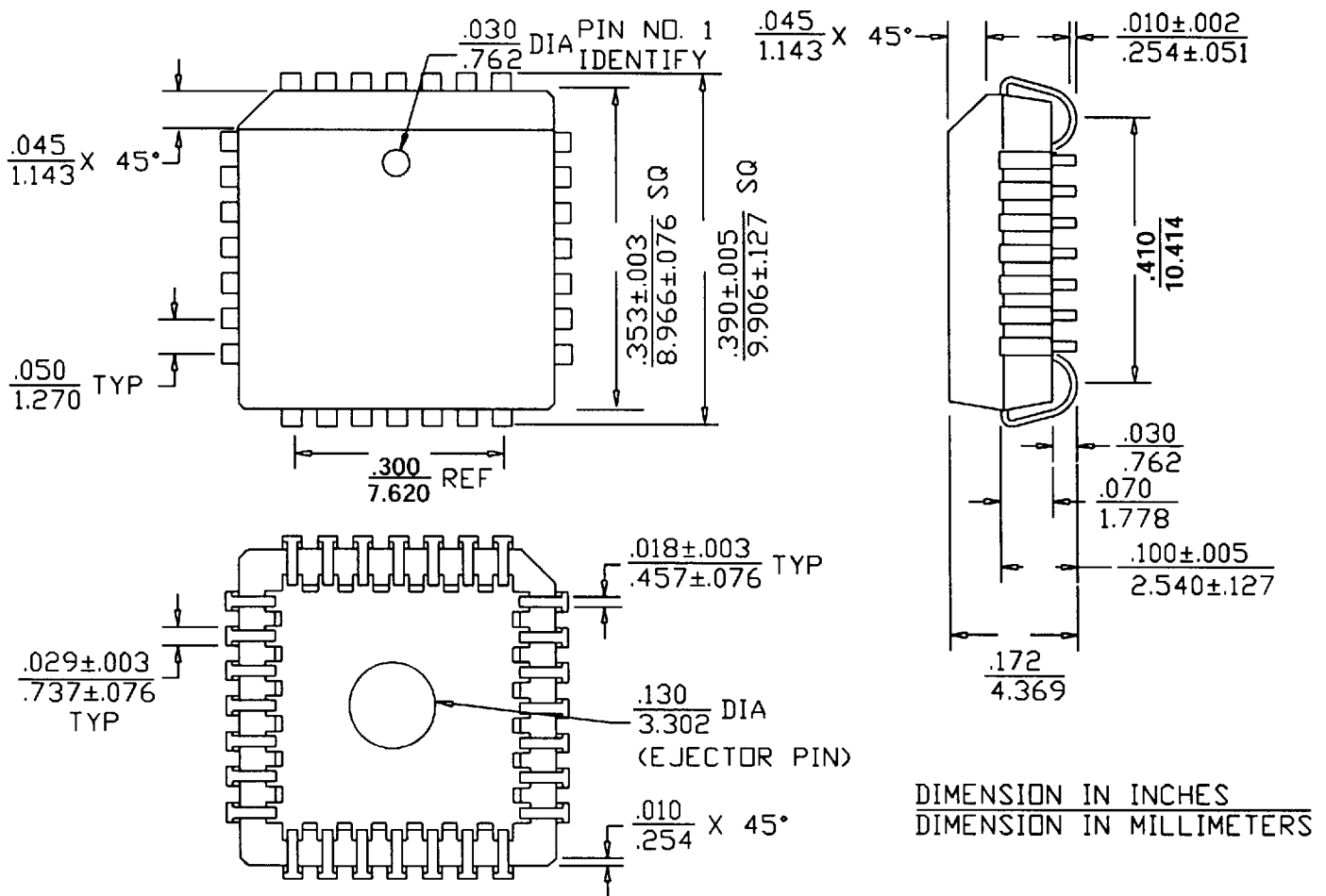
28-Pin PLCC (J28)
