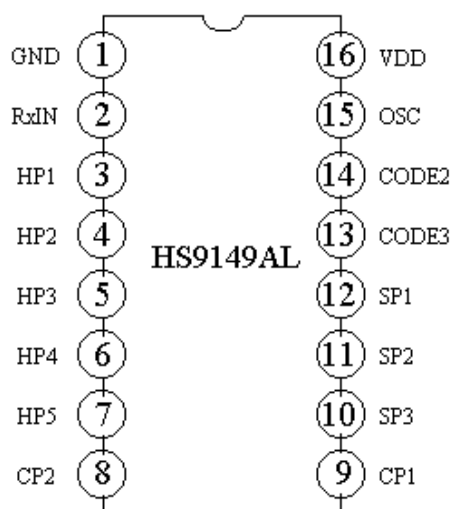
管脚图
