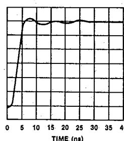
PULSE RESPONSE 10 VOLT STEP
