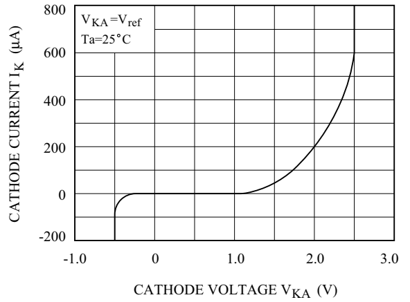
I_K - V_{KA}
