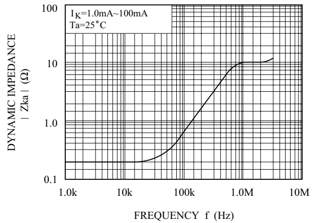
|Z_{ka}| - f
