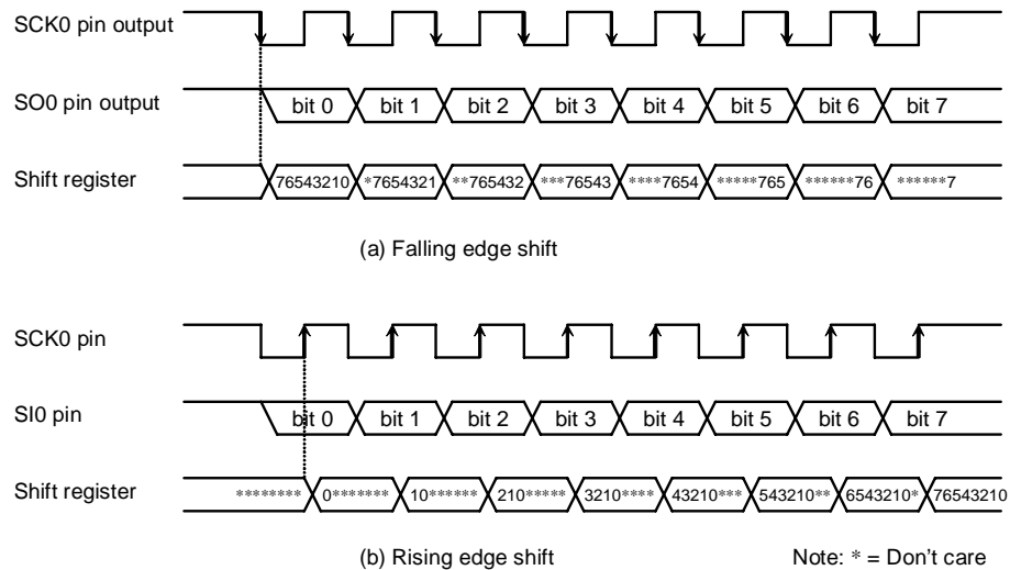
Figure 3.10.38 Shift Edge
