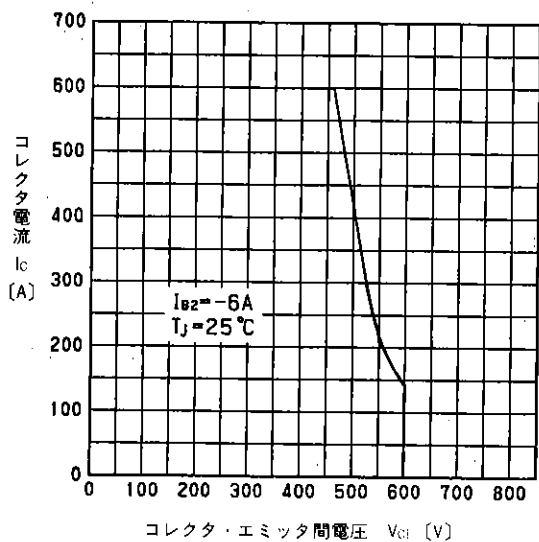
安全動作領域(逆バイアス) RRReverse Bias Safe Operating Area
