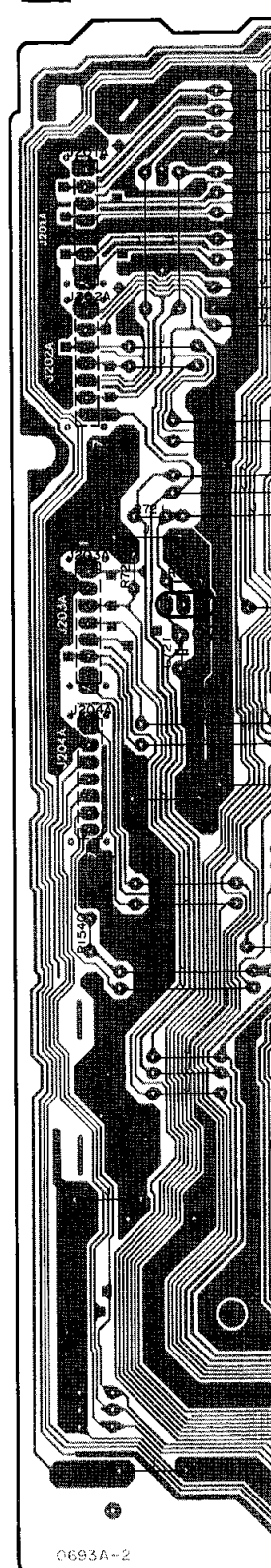
G MAIN P.C.B.
