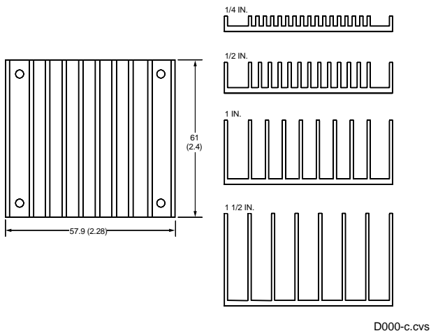
Figure 35. Longitudinal Heat Sink
