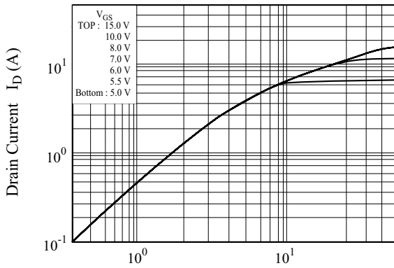
I_D - V_{DS}
