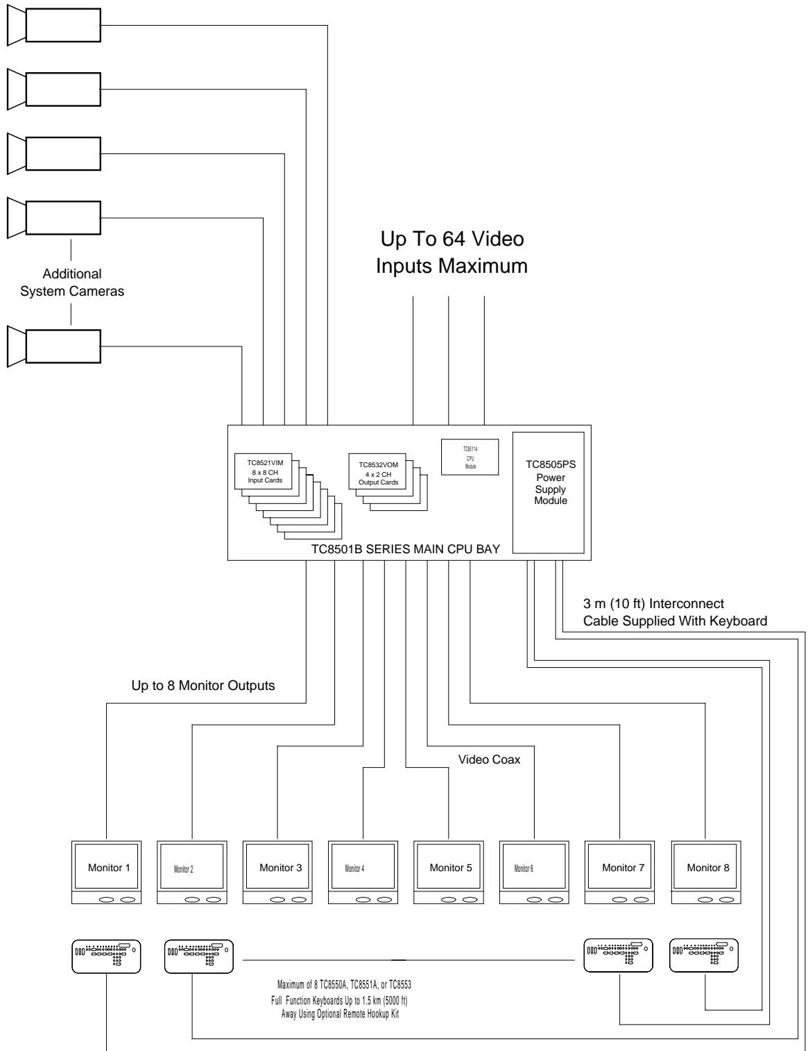
Sistema de conmutación de video TC8500
