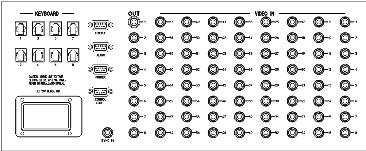
Ilustración del Tablero Trasero Serie TC8501
