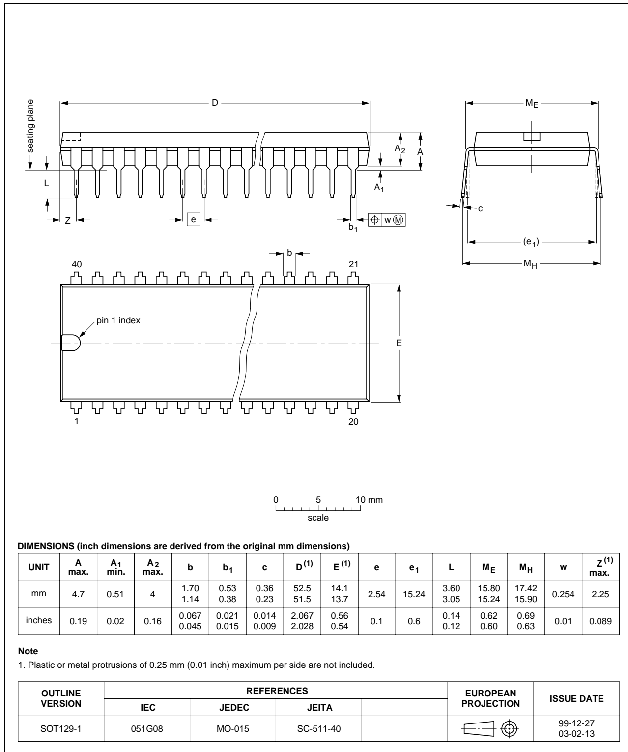
Fig 27. DIP40 (SOT129-1).
