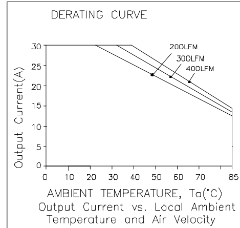
V_{in}=12\text{ V} , V_o=1.8\text{ V}
