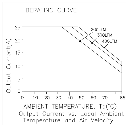
V_{in}=12\text{ V} , V_o=3.3\text{ V}
