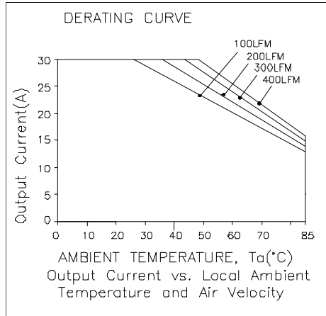
V_{in}=12\text{ V} , V_o=0.8\text{ V}
