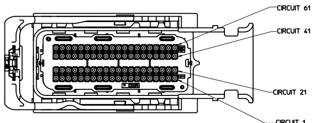
80 CKT
