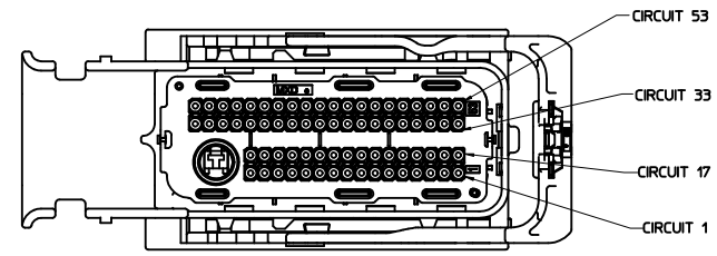
73 CKT
