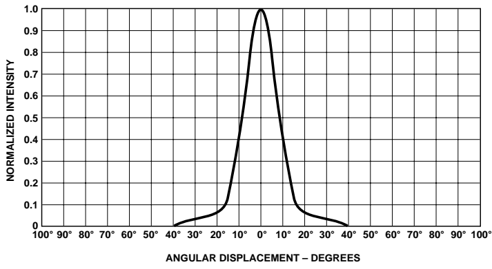
Figure 8. HLMP-Q106/-Q156.
