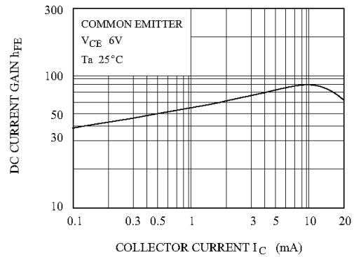
h_{FE} - I_C
