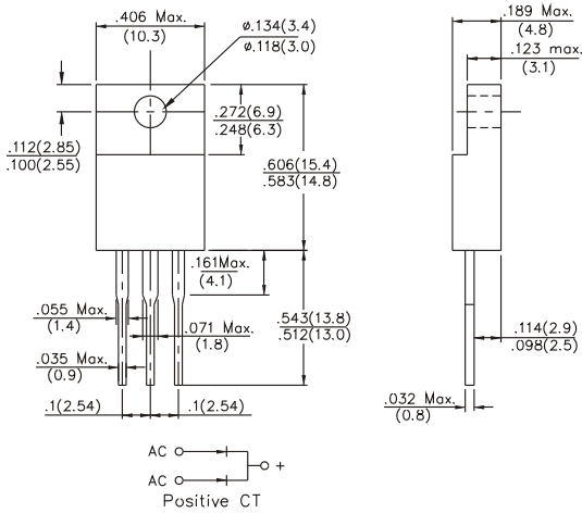
ITO-220AB
