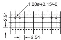
CTDD2709SF-D1K-2 Footprint
