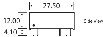
CTDD2709SF-D1K-2 Package
