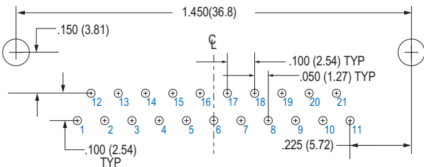
21 SOCKET M83513/19-C
