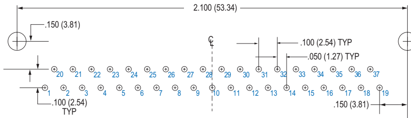
37 SOCKET M83513/19-F
