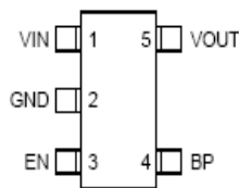
SOT-23-5
