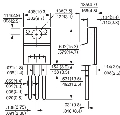
ITO-220
