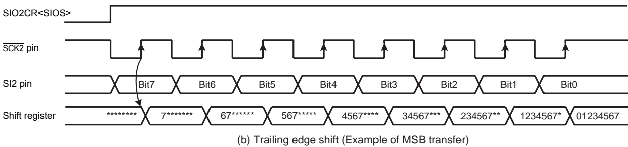
Figure 15-4 Shift Edge
