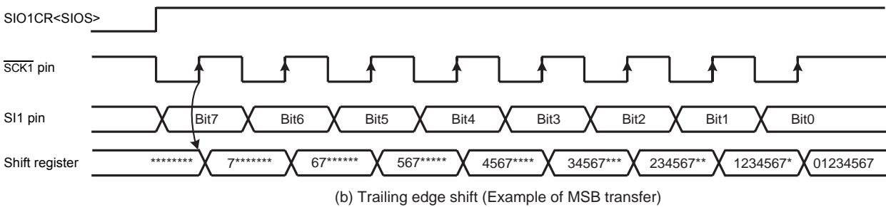
Figure 14-4 Shift Edge
