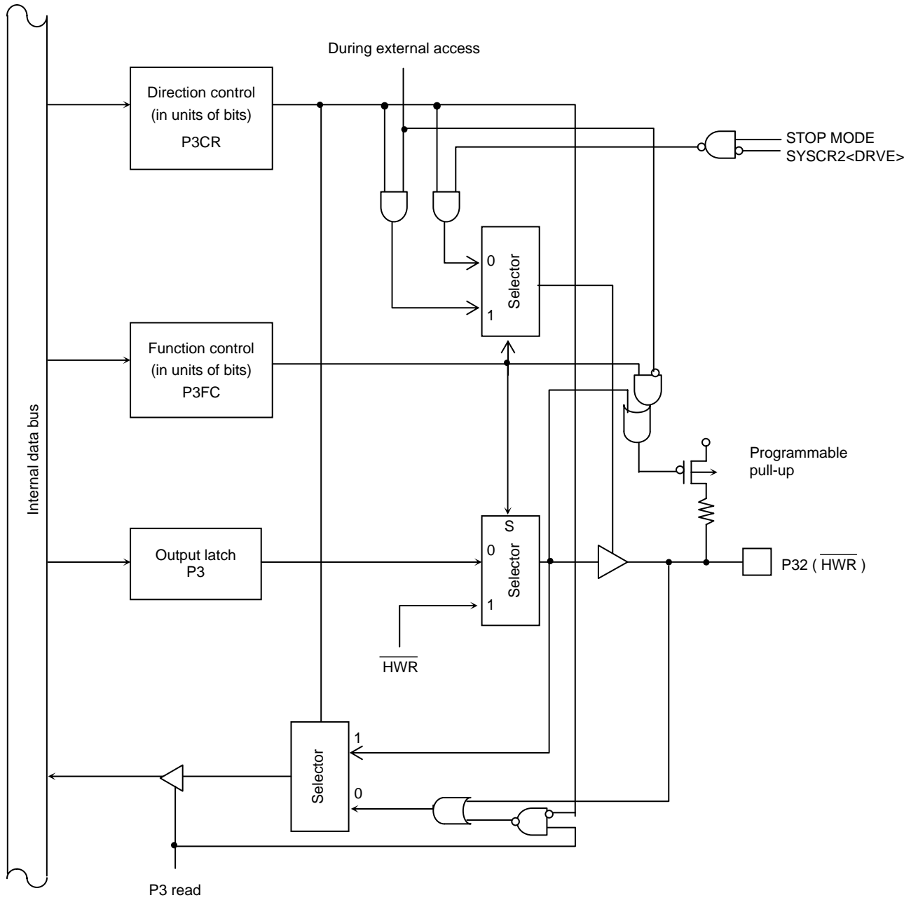
Fig. 7.4.2 Port 3 (P32)
