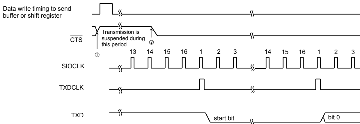
Fig. 13.3.9.1 Handshake Function
