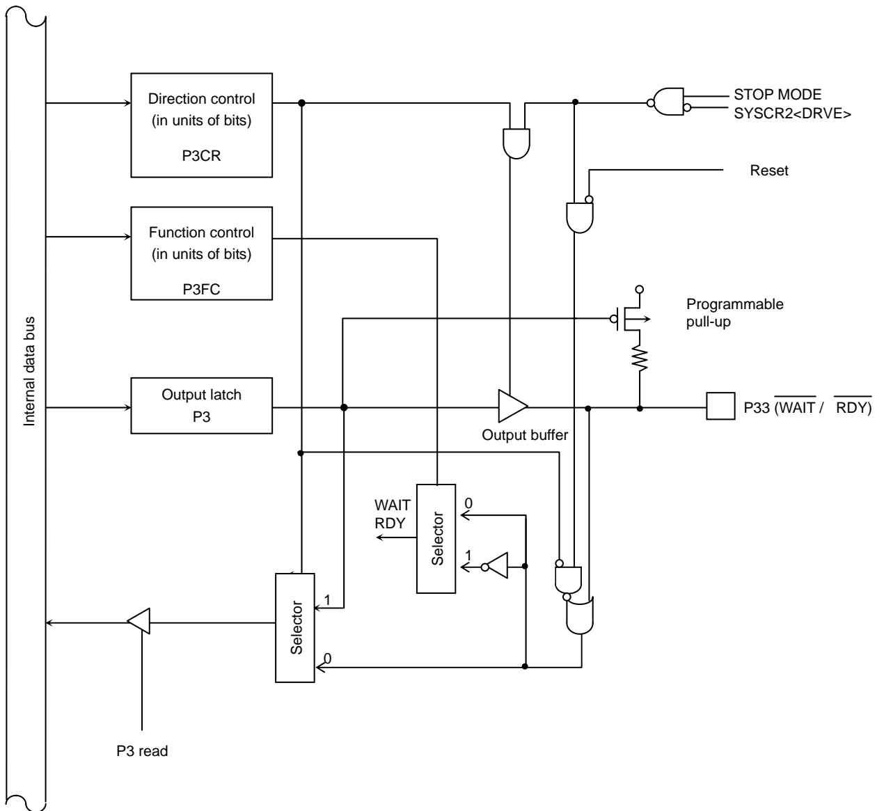
Fig. 7.4.3 Port 3 (P33)
