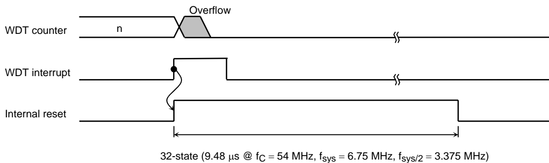
Fig. 16.2.2 Reset Mode
