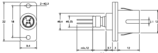
SC Receptacle
