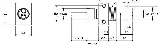
ST Receptacle
