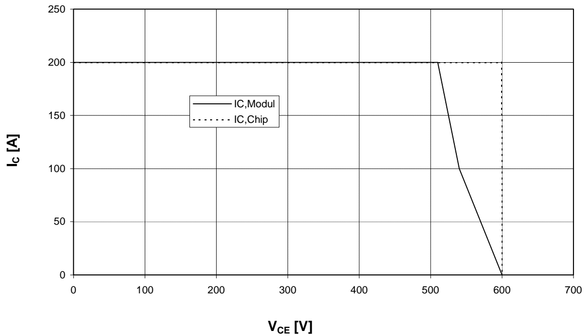
Sicherer Arbeitsbereich Wechsell. (RBSOA) I_C = f(V_{CE}) Reverse bias safe operating area Inverter (RBSOA) T_{vj} = 125^\circ\text{C} , V_{GE} = \pm 15\text{V} , R_G = 15 \text{ Ohm}
