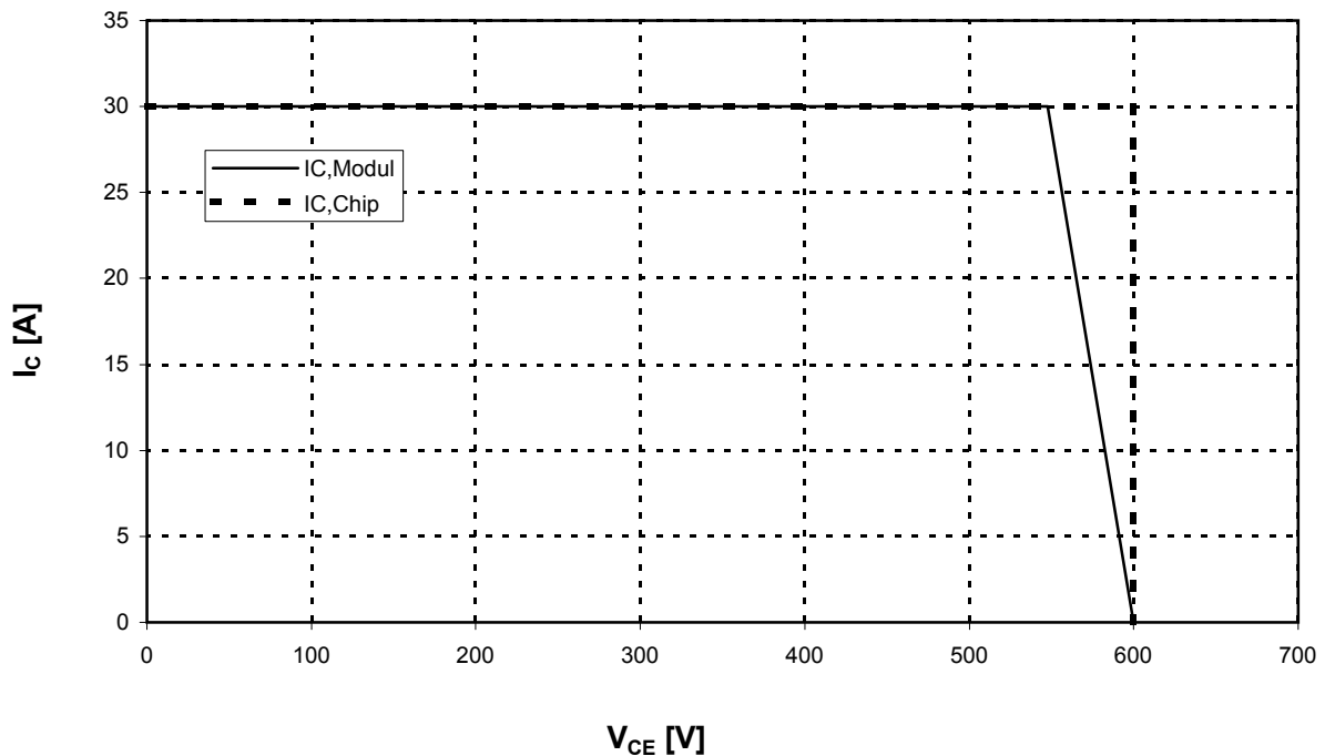
Sicherer Arbeitsbereich Wechsler. (RBSOA) I_C = f(V_{CE}) Reverse bias safe operating area Inverter (RBSOA) T_{vj} = 125^\circ\text{C} , V_{GE} = \pm 15\text{V} , R_G = 68 \text{ Ohm}
