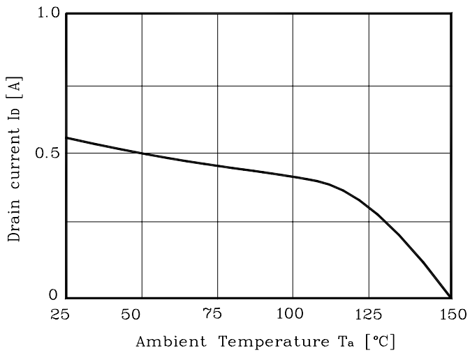
Fig. 9 I_D - T_a
