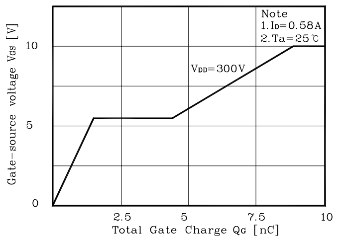
Fig. 6 V_{GS} - Q_G
