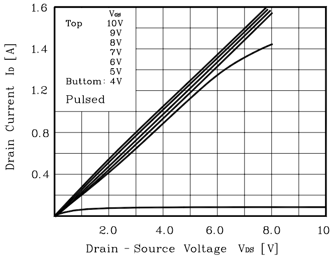
Fig. 1 I_D - V_{DS}
