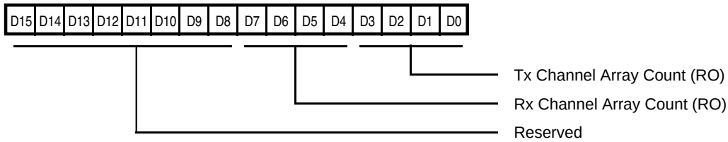
Figure 13a. DMA Array Count Register (DACR)
