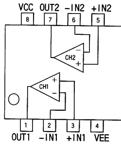
F:SOP8 FV:SSOP-B8 FVM:MSOP8
