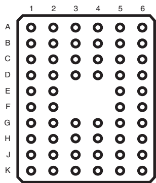
56-Ball BGA
