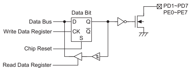
PD1~PD7, PE Output Ports
