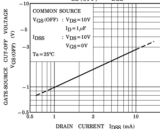
V_{GS(OFF)} - I_{DSS}
