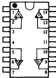
NJM2058D NJM2058M NJM2058L
