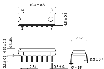
DIP14
