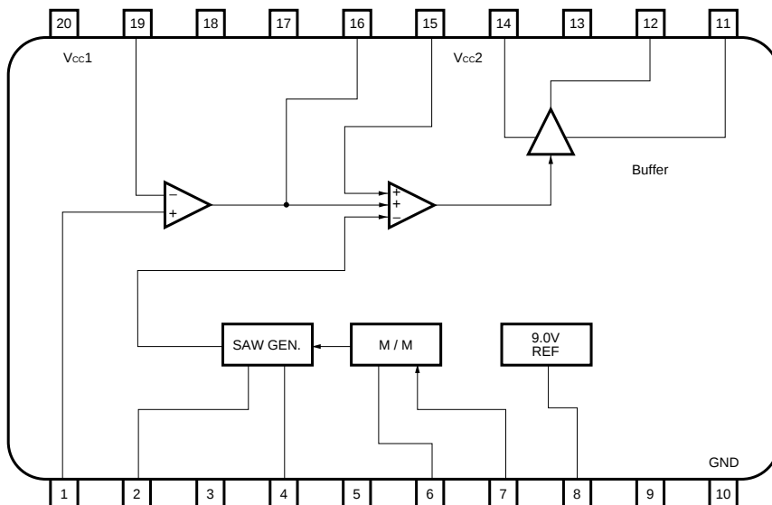
BA9756FS
