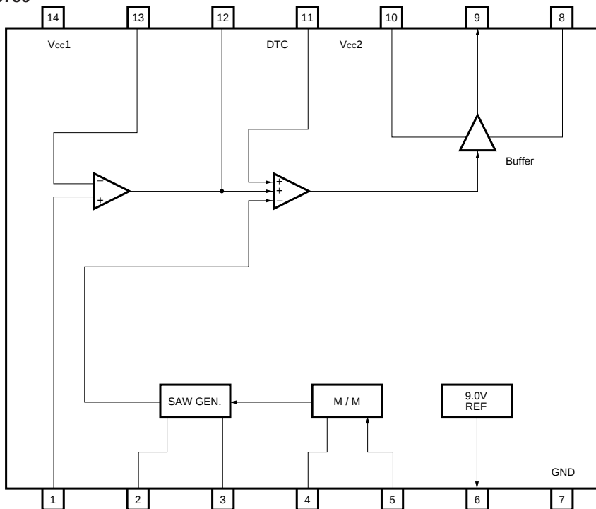
BA9756
