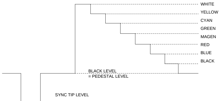
Fig. 8 YOUT output
