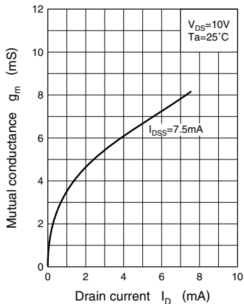
g_m - I_D
