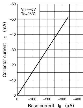
I_C - I_B
