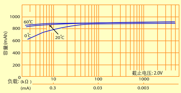
容量、负载特性
