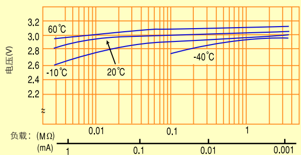
工作电压、负载特性
