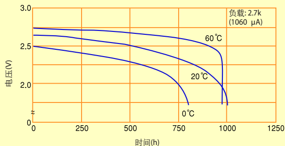
温度特性
