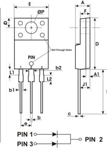
ITO-220AB
