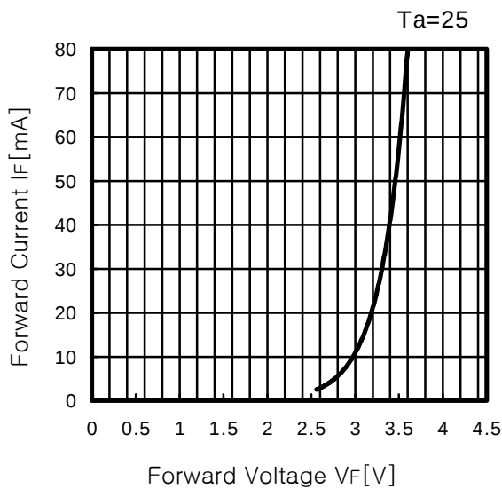
Fig. 1 I_F - V_F
