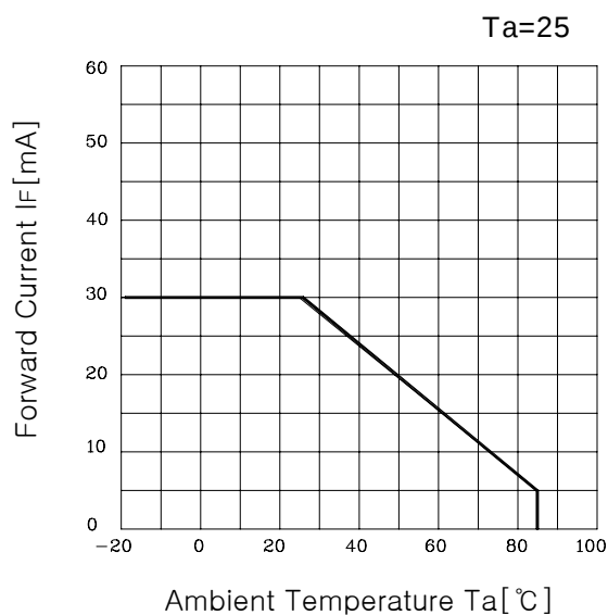
Fig. 3 I_F - T_a
