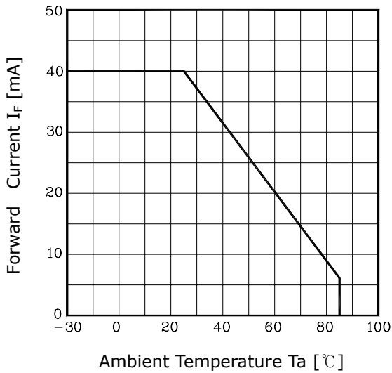
Fig. 3 I_F - T_a
