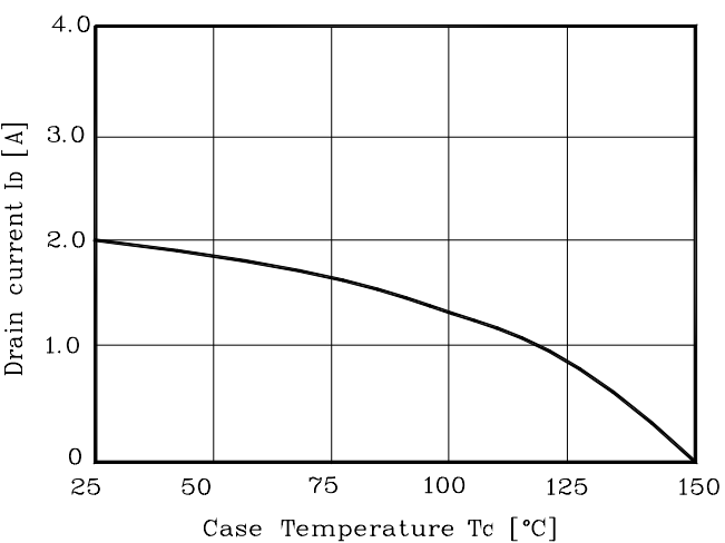
Fig. 9 I_D - T_C
