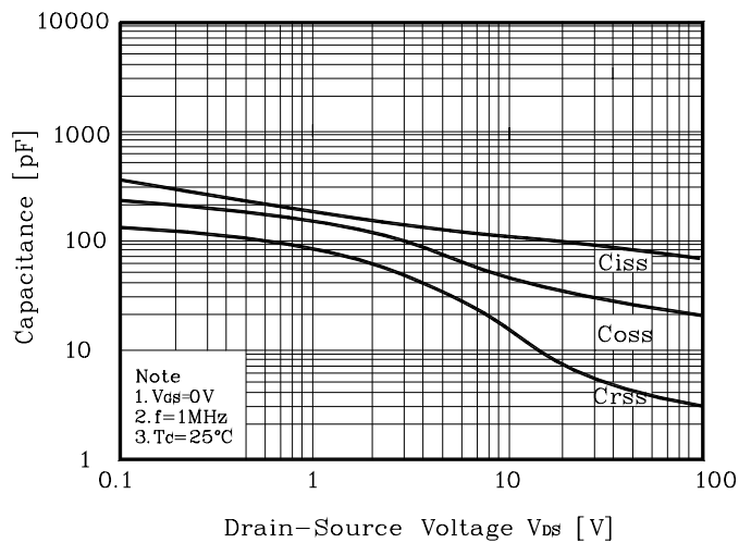
Fig. 5 Capacitance - V_{DS}
