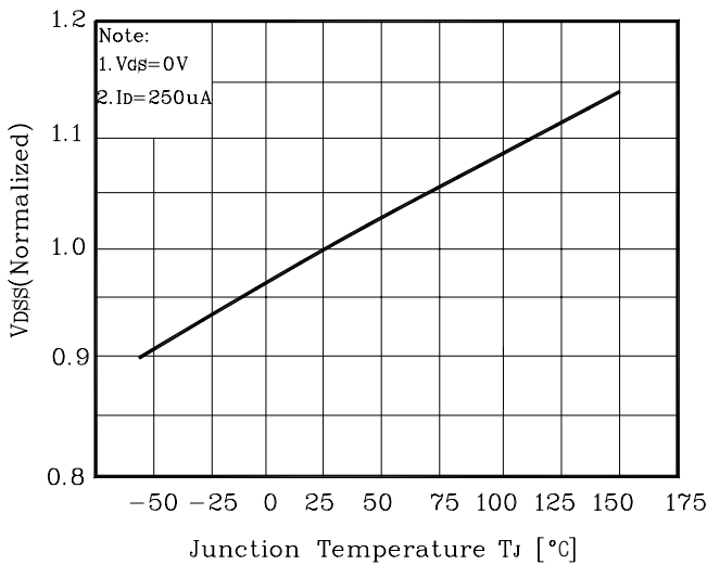
Fig. 7 V_{DS} - T_J
