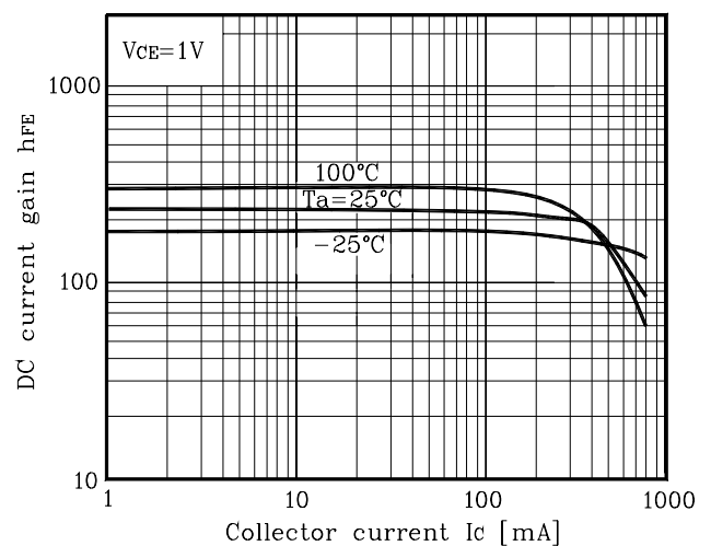
Fig. 6 h_{FE} - I_c
