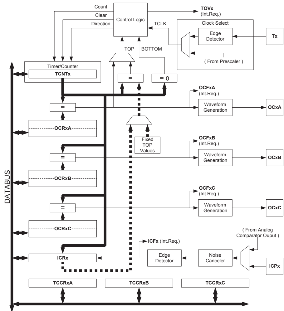
Figure 46. 16 位 T/C 框图
