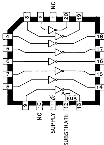
UDN-2580/85EP
