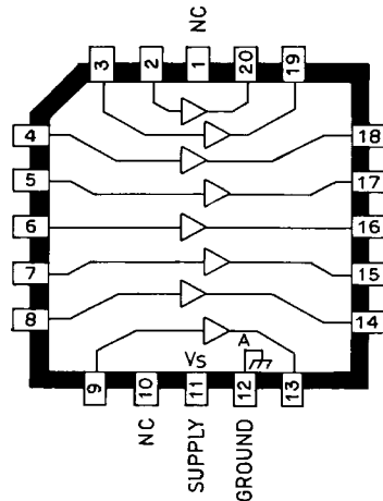
UDN-2982/84EP UDS-2982/84EK
