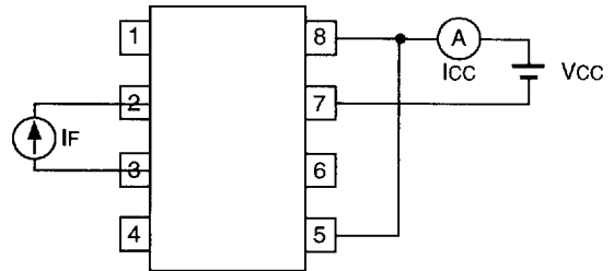
FIG. 6 (IcCL, IcCH)
