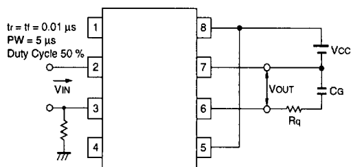
FIG. 8 (tPLH, tPHL)
