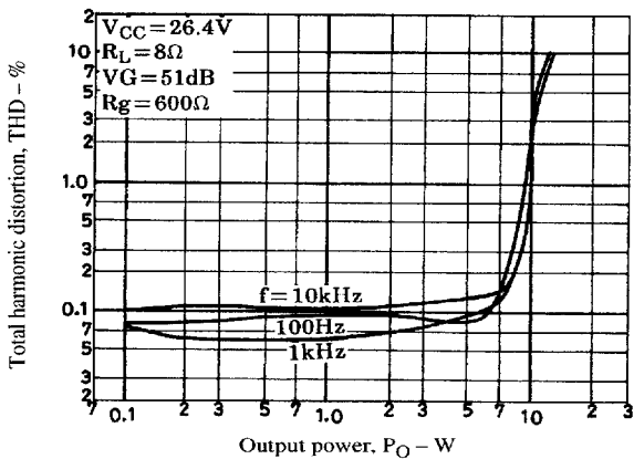
THD - P_O
