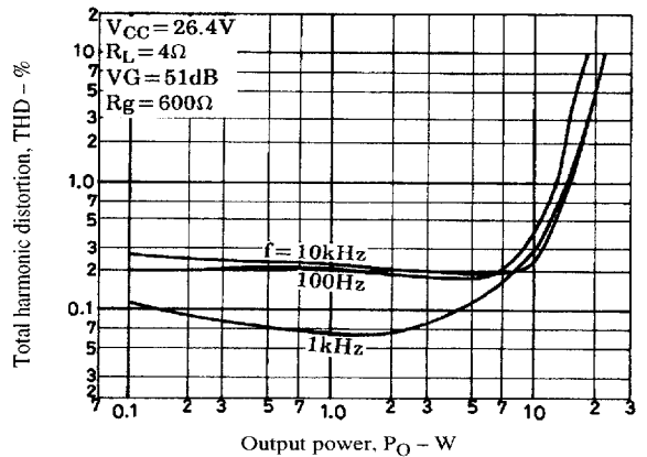
THD - P_O
