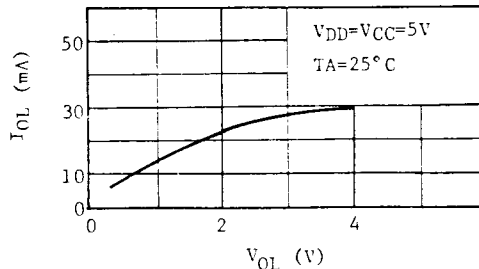
3) BUS, P1, P2: I_{OL} - V_{OL}
