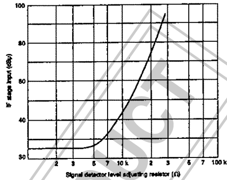
Figure 16. IF input vs. R_{SD \text{ de } j}
